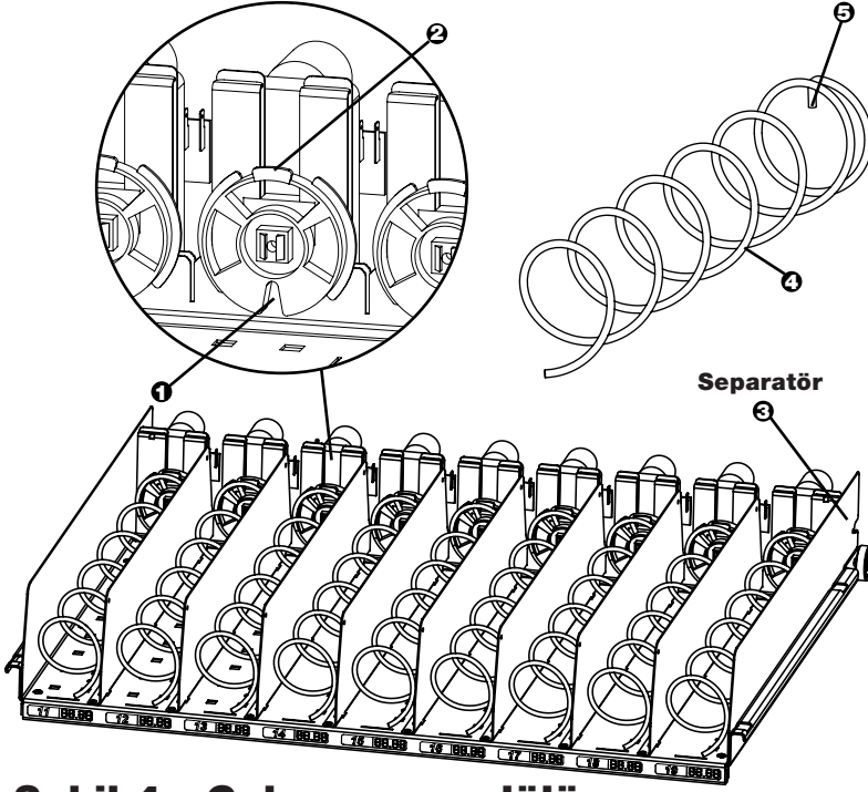
Şekil 4 - Çekmece modülü
