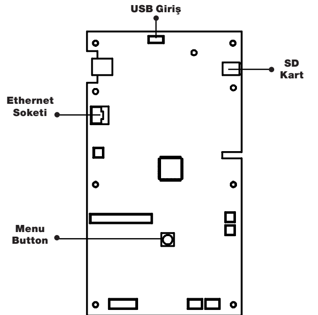
Anakart Modülü
